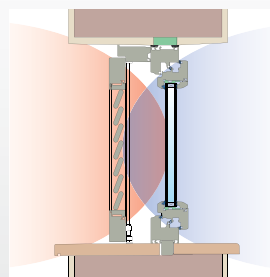
aislamiento térmico en verano
