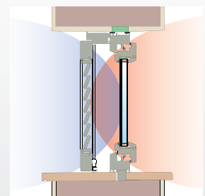
aislamiento térmico en invierno
