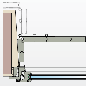
montaje sobre marco
