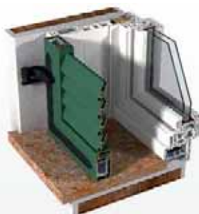
renovación con marco D 352
